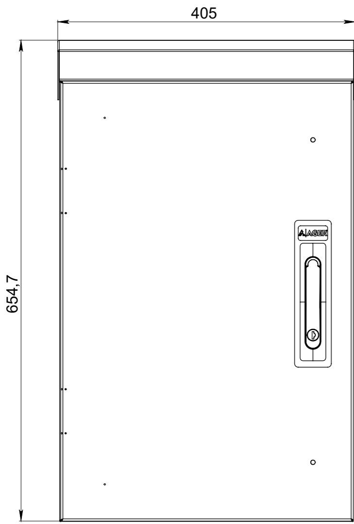
Ön Görünüş
