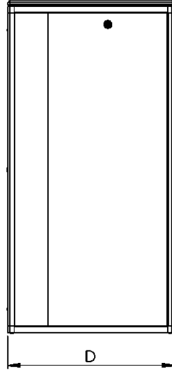
Yan Görünüş
